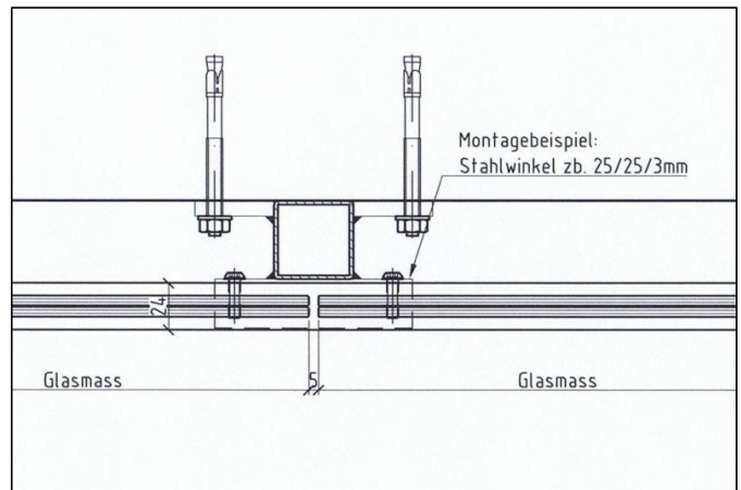
Horizontal bei Rohr-Pfosten:
