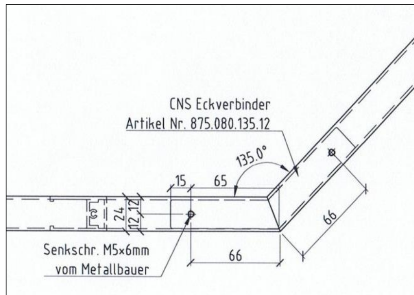
Draufsicht 135° Eckverbinder Verbohrung
