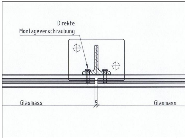
Horizontal bei T-Pfosten:
